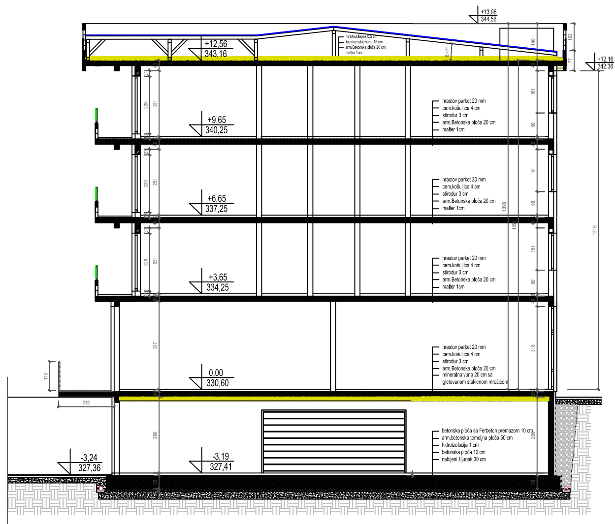
PRESEK B-B
