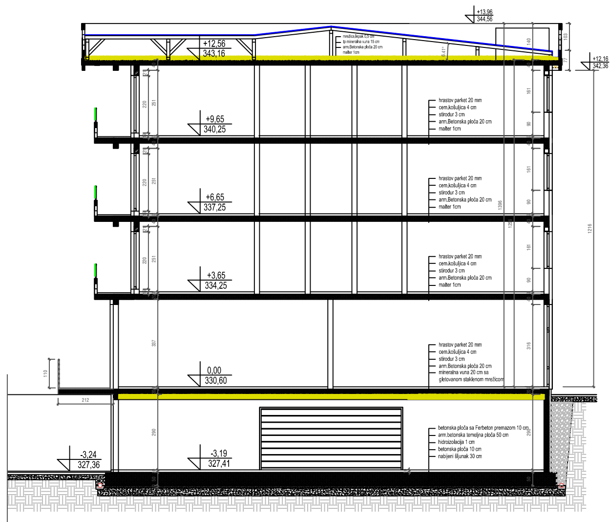
PRESEK B-B
