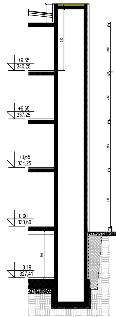
Detalj preseka lift okna
